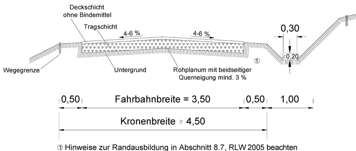
Abbildung 2: Querschnitt Holzabfuhrweg im "Dachprofil"
