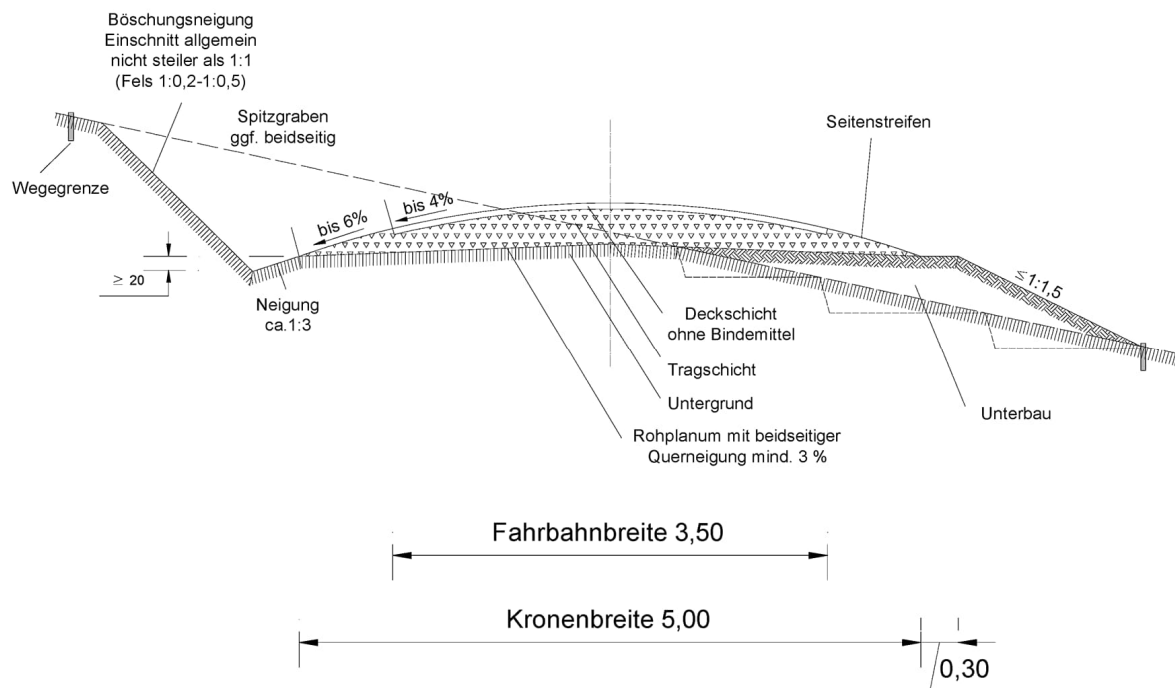
Abbildung 1: Querschnitt Holzabfuhrweg im "Uhrglasprofil"
