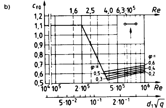
Bild 7. Grundkraftbeiwerte c_{f0} für ebene Fachwerke aus Kreiszyylinderrohren in Abhängigkeit von der Reynoldszahl Re^3
