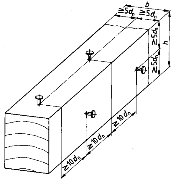
Bild A.1. Prüfkörper aus Fichte
