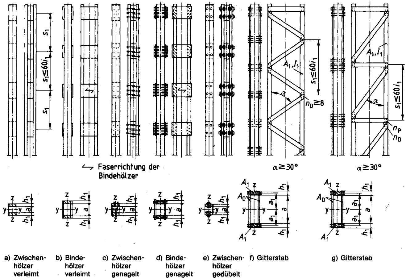
Bild 22. Bauarten von Rahmen- (a bis e) und Gitterstäben (f und g)
