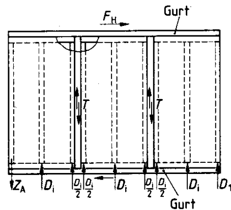
b) Aus Einraster-Tafeln zusammengefügte Tafeln; Z_A , D_1 und Schnittkraft T
