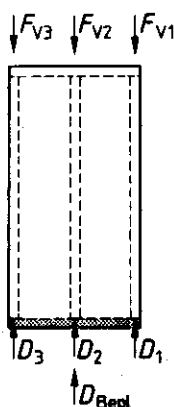
Bild 35. Einraster-Tafel unter lotrechten Lasten F_{Vi} , Rippen-Druckkräfte D_i im Schwellenbereich und Anschlußkraft D_{\text{Bepl}} der Beplankung an die Schwelle
