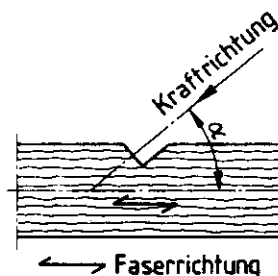
Bild 2. Krafftrichtung schräg zur Faserrichtung
