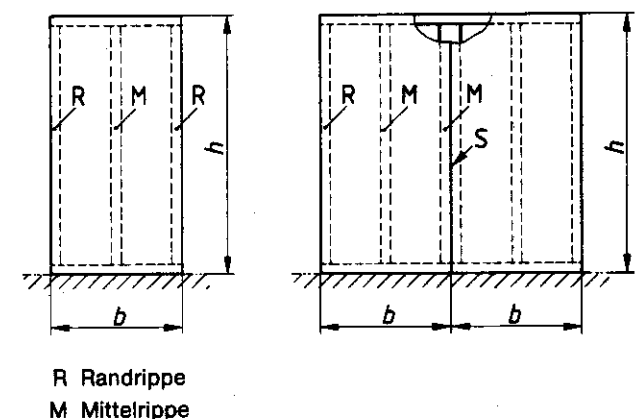
Bild 31. Beispiele für Einraster- und Mehr raster-Tafeln
