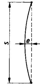
Bild 24. Stab mit ungewollter Ausmitte e im unbelasteten Zustand
