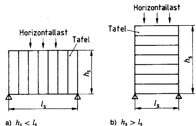
Bild 30. Beispiele für Dach- oder Deckenscheiben aus Tafeln (Draufsicht); Maße, Last
