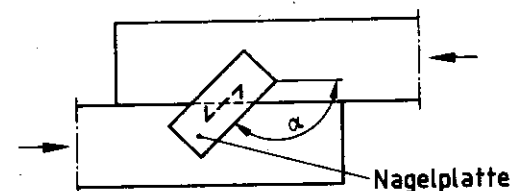
b) Druckscheren ( 90^\circ < \alpha < 180^\circ )
