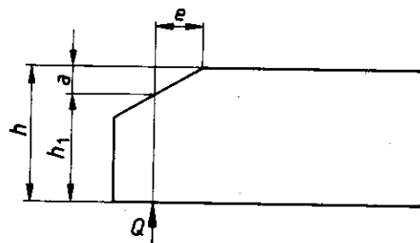
b) Abschrägung
