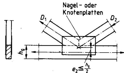
b) bei Bindern mit Nagel- oder Knotenplatten
