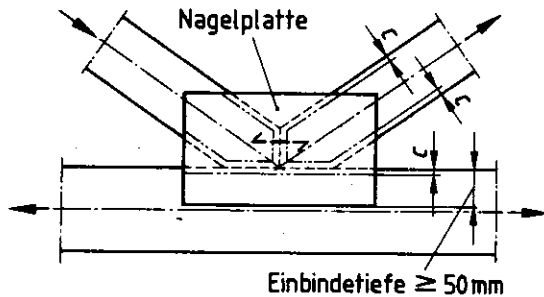
a) Beispiel eines Knotenpunktes
