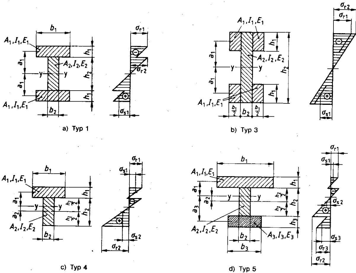
Bild 15. Verschiedene Querschnittstypen zusammengesetzter Biegeträger und Spannungsverteilung (schematisch) bei positivem Biegemoment
