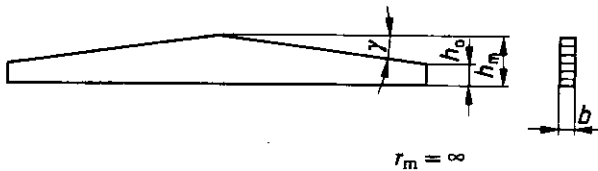
Bild 12. Satteldachträger mit geradem Untergurt
