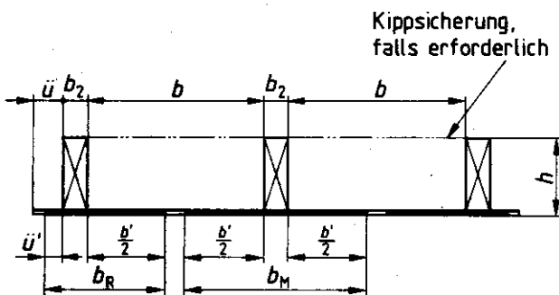
b) einseitige Beplankung
