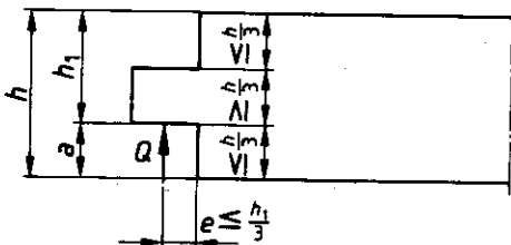
b) Rechteckige Ausklinkung mit Verstärkung
