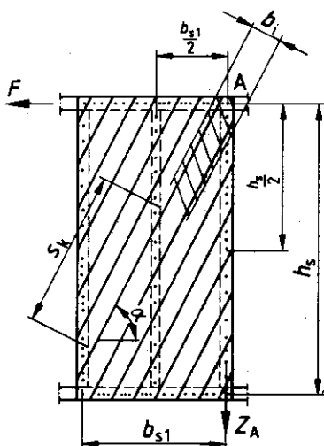
Bild 1. Wandtafeln mit diagonalen Bretterschalung (Einraster-Tafel)
