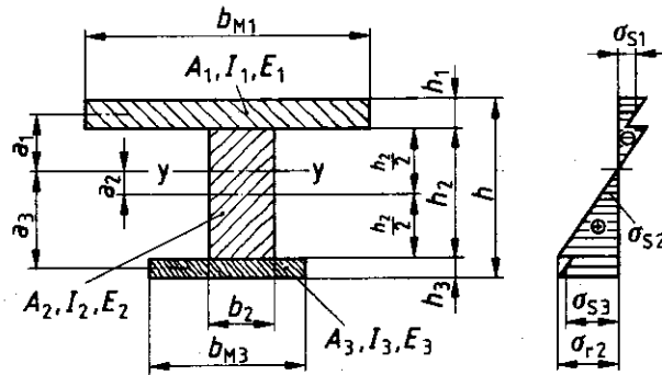
Bild 29. Unsymmetrischer Querschnitt mit beidseitiger Beplankung
