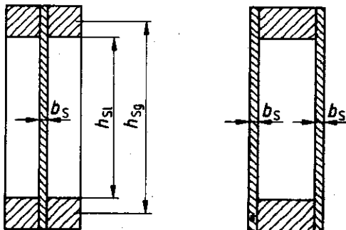
a) I-Querschnitt
