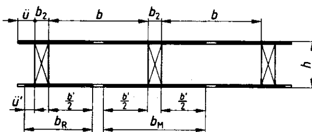
a) beidseitige Beplankung
