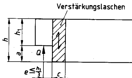
b) Rechteckige Ausklinkung mit Verstärkung
