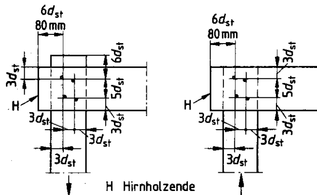
Bild 11. Mindestabstände bei Stabdübeln und Paßbolzen
