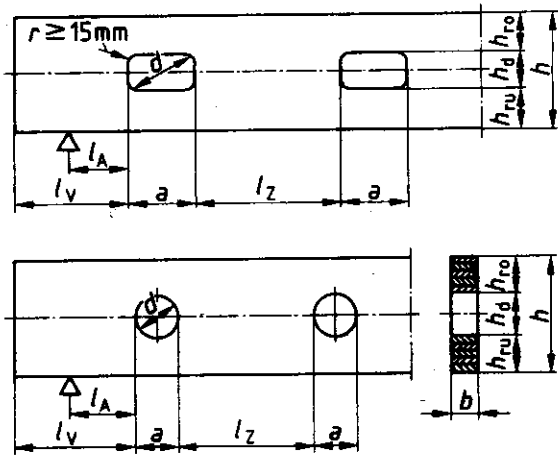
Bild 8. Maße und Anordnung von Durchbrüchen
