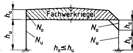
Bild 19. Zweigelenkrahmen mit Fachwerkgiebel
