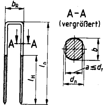
Bild 20. Tragende Klammer
