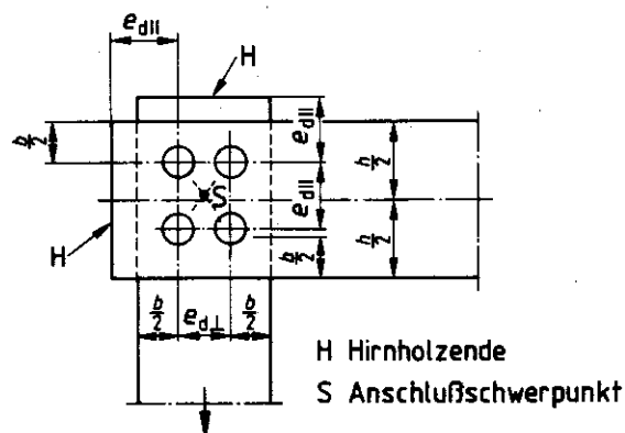
Bild 10. Mindestdübelabstände bei Queranschlüssen
