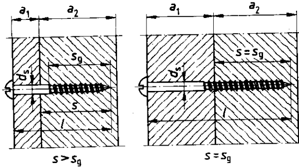
Bild 21. Holzplatten und Einschraubtiefen bei Holzschrauben
