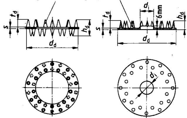
a) zweiseitiger Dübel
