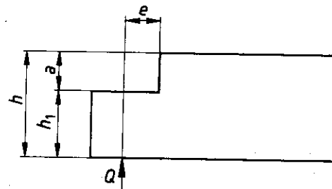
a) Rechteckige Ausklinkung
