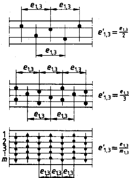
Bild 16. Maßgebender Abstand e'_{1,3} bei mehrreihiger Anordnung der Verbindungsmittel
