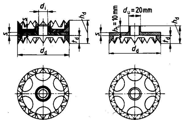
a) zweiseitiger Dübel
