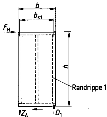
Bild 32. Anker-Zugkraft Z_A und Druckkraft D_1 im Schwellenbereich
