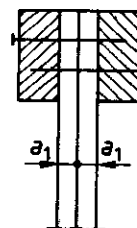
Bild 14. Zweischnittige Gurtanagelung bei Vollwandträgern
