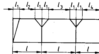
Bild 14. Feldweiten bei Kopfbandbalken
