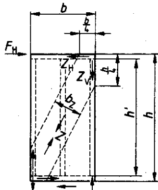
Bild 33. Verteilung und Anschluß der Streben-Zugkraft Z bei einseitiger Beplankung
