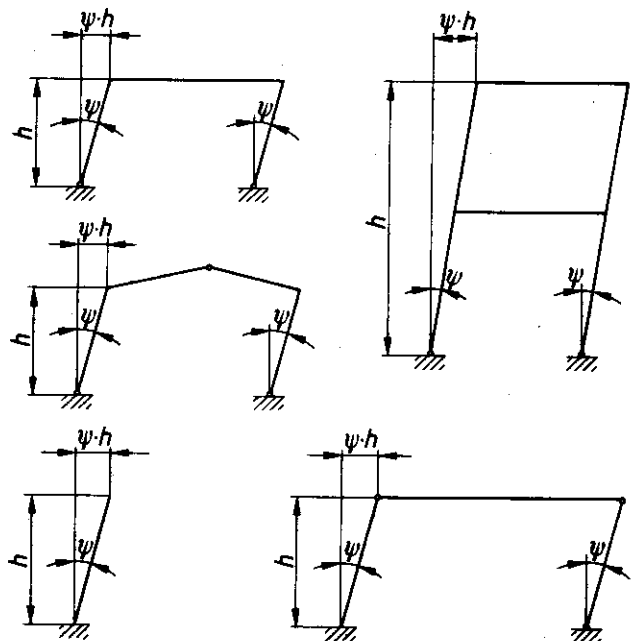
Bild 25. Rahmensysteme, Einzelstützen und Stützenreihen mit ungewollter Schrägstellung der Stiele
