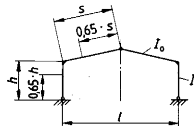
Bild 21. Rahmensystem
