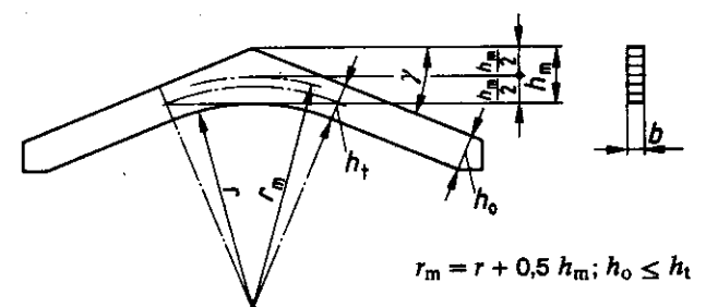
Bild 11. Satteldachträger mit gekrümmtem Untergurt
