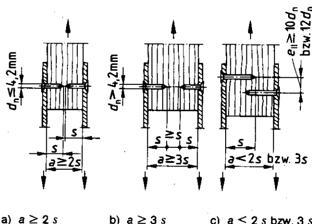
Bild 19. Holzdecken bei Stahlblech-Holz-Nagelung ohne versetzte Anordnung benachbarter Nägel
