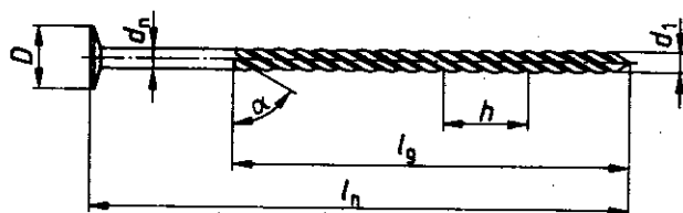
a) Schraubnagel
