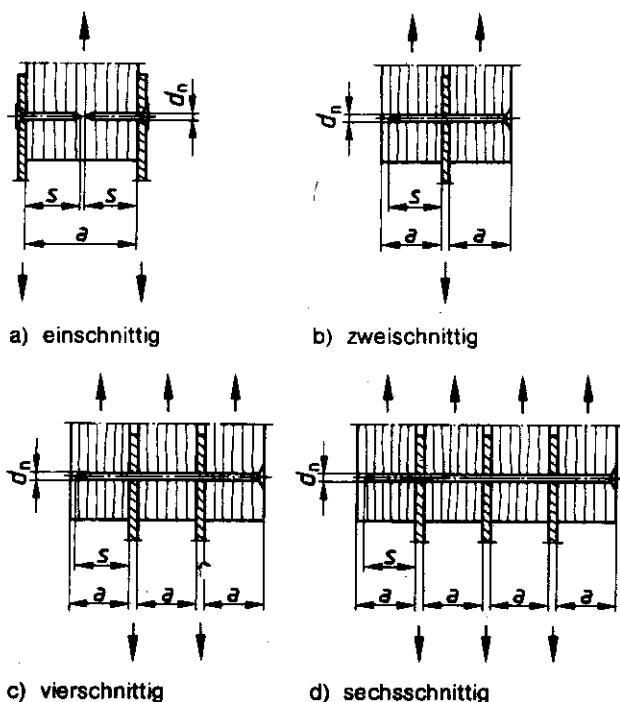
Bild 18. Holzdecken und Einschlagtiefen bei Stahlblech-Holzverbindungen
