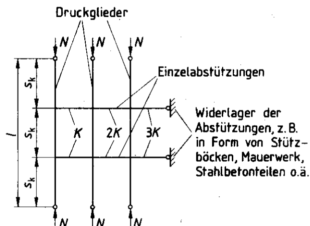
Bild 27. Einzelabstützung von Druckgliedern
