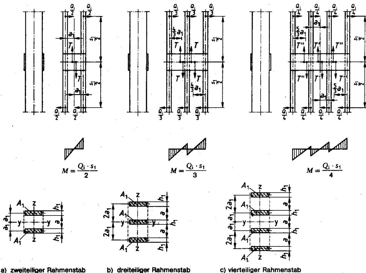
Bild 23. Annahmen über die Angriffspunkte der Quer- und Schubkräfte bei mehrteiligen Rahmenstäben (Beispiel: Rahmenstäbe mit Bindehölzern)
