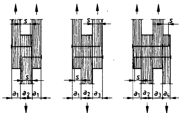
a) einschnittig b) zweischnittig c) dreischnittig
