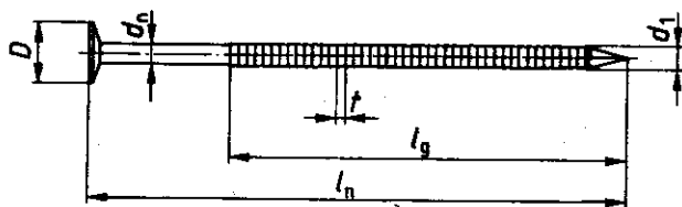
b) Rillennagel
