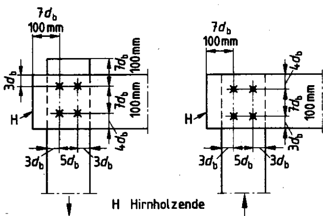
Bild 12. Mindestabstände bei tragenden Bolzen
