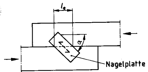
a) Zugscheren ( \alpha < 90^\circ )
