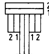
Bild 18. Zusammengesetzter Gurtquerschnitt eines genagelten Vollwandträgers
