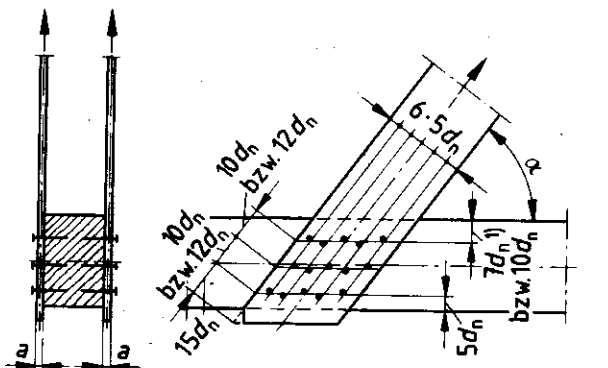
a) einschnittige Nagelung
