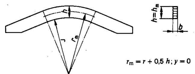
Bild 10. Gekrümmter Träger mit konstanter Trägerhöhe
