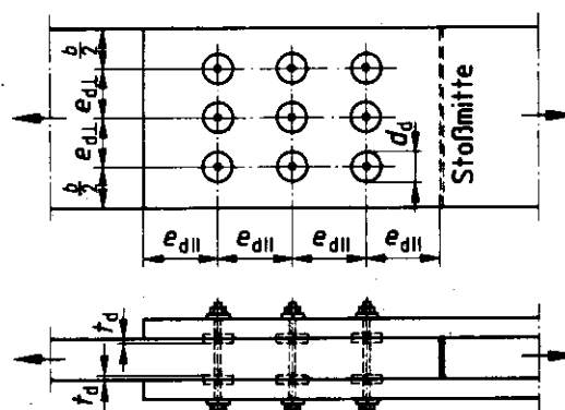
a) nicht versetzte Anordnung
