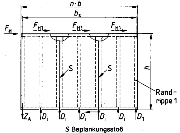
a) Anker-Zugkraft Z_A und Rippen-Druckkräfte D_1 im Schwellenbereich
