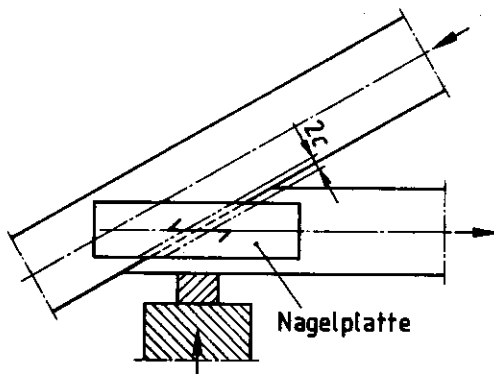
b) Beispiel eines Traufpunktes
