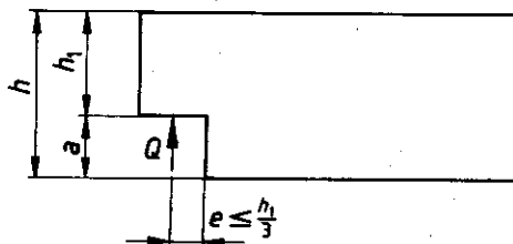
a) Rechteckige Ausklinkung ohne Verstärkung
