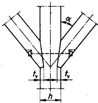
Bild 25. Zweiseitiger Versatzeinschnitt
