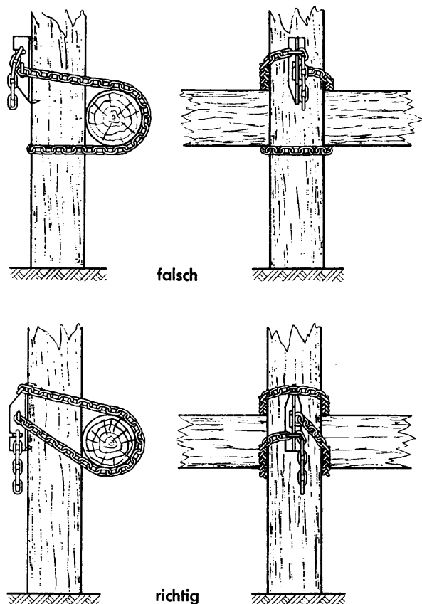
Bild 4 Kettenbindung mit dem ⊥-Eisenschloß
