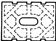
Bild 3 Kalksand-Lochstein Zweieinviertelnormalformat (Die dargestellte Lochung ist nur ein Beispiel)
