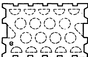
Bild 4 Kalksand-Hohlblockstein (Die dargestellte Lochung ist nur ein Beispiel)
