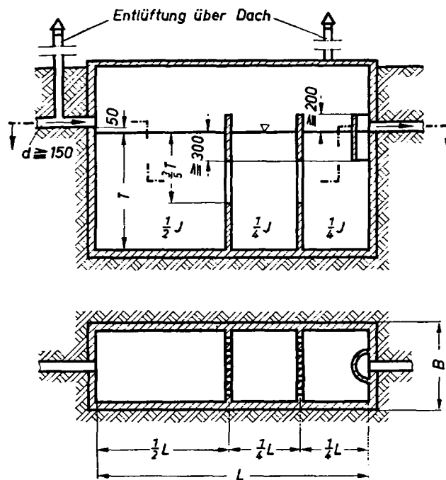
Bild 2 Dreikammer-Grube (längs durchflossen)
