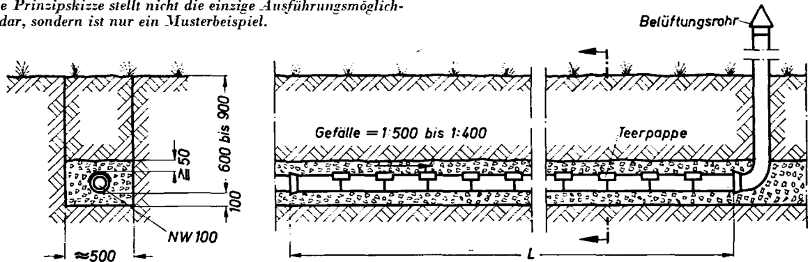
Bild 5a Rieselrohr-Graben
