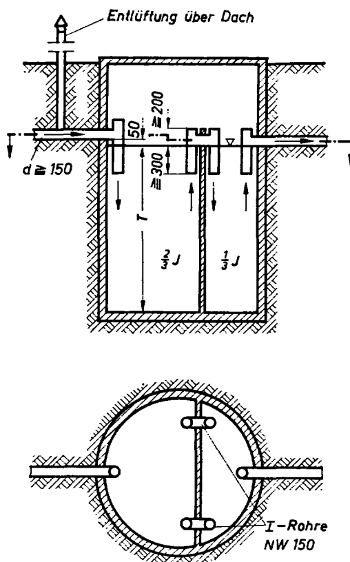
Bild 1 Zweikammer-Faulgrube (senkrecht durchflossen)
