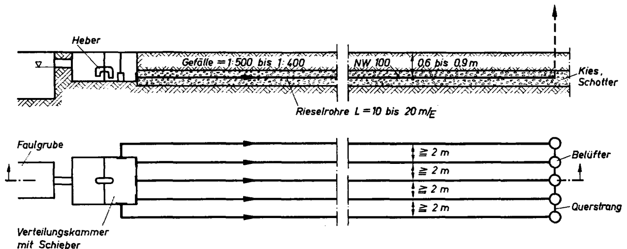
Bild 5b Rieselrohr-Netz
