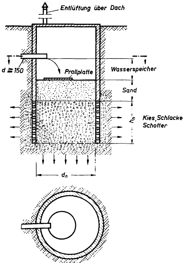
Bild 6 Sickerschacht
