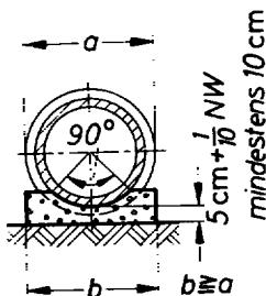
Rohr satt auf Beton aufliegend
