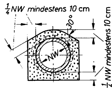
Bild 12. Ausführungsbeispiel einer vollen Ummantelung mit Beton
