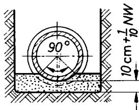
Sandbett sorgfältig verdichtet
