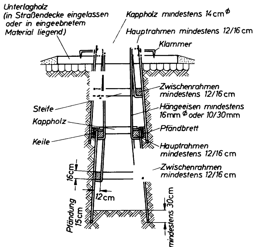
Bild 4. Ausführungsbeispiel eines waagerechten Verbaus
