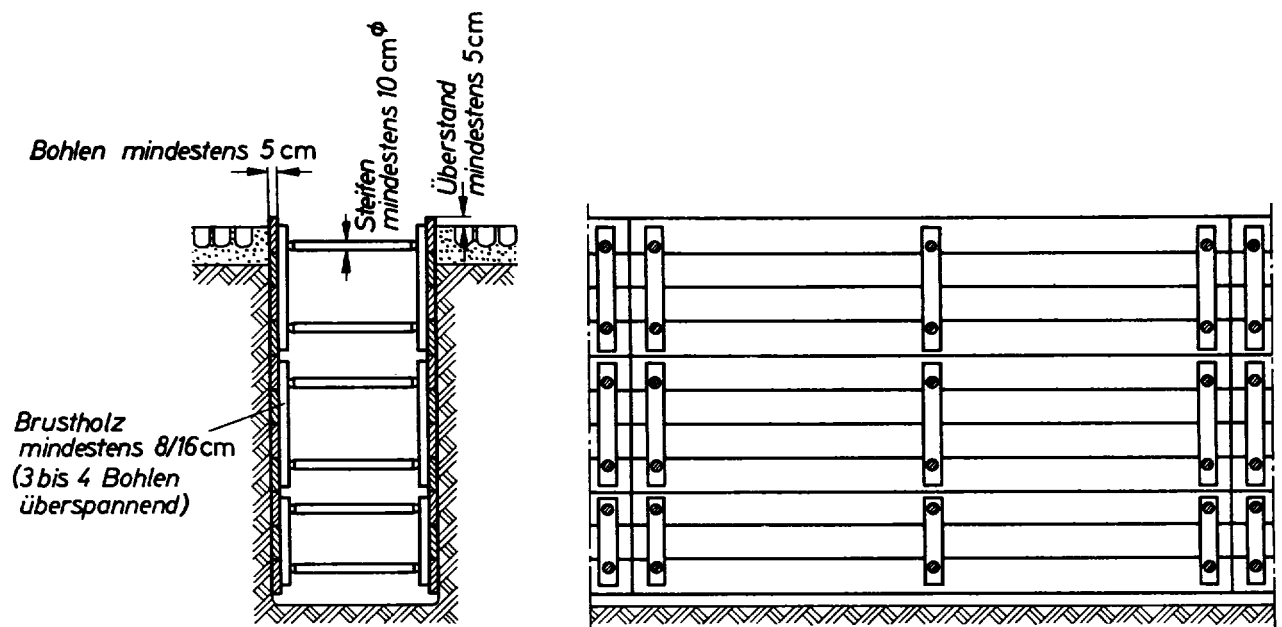
Bild 4. Ausführungsbeispiel eines waagerechten Verbaus
