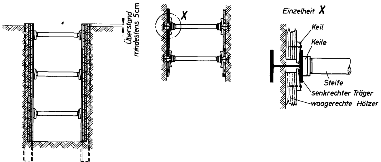
Bild 6. Ausführungsbeispiel eines Verbaus mit Bohlen zwischen geramten oder in Bohrlöcher eingebrachten Trägern
