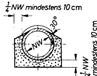
Bild 11. Ausführungsbeispiel einer Teilummantelung mit Beton
