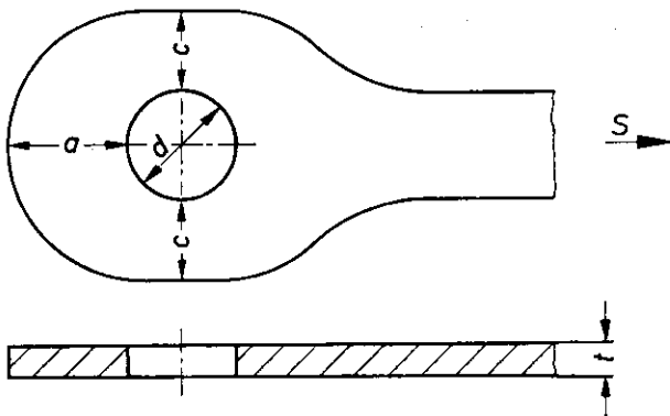
Bild 9. Bezeichnungen bei Augenstäben
