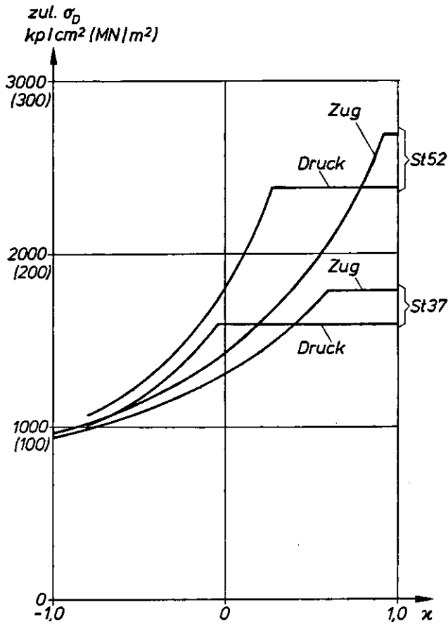
Bild 5. Zulässige Spannung für die Dauerfestigkeit; Kerbfall 1
