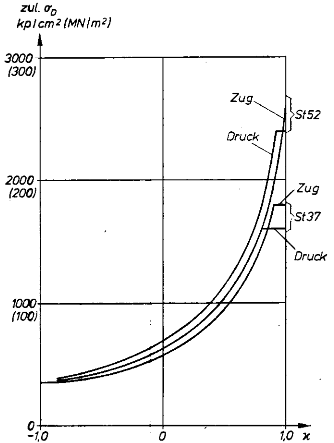
Bild 8. Zulässige Spannung für die Dauerfestigkeit; Kerbfall 4
