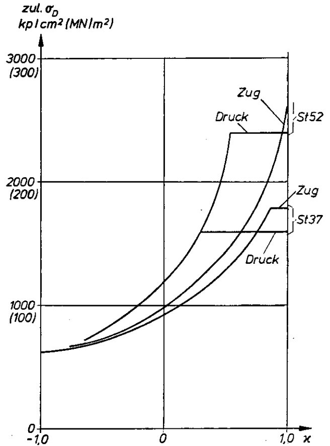
Bild 6. Zulässige Spannung für die Dauerfestigkeit; Kerbfall 2
