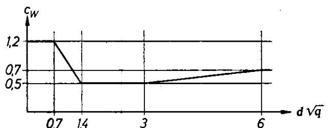
Bild 2. Darstellung des Formbeiwertes c_W für zylindrische Baukörper in Abhängigkeit von d \cdot \sqrt{q} für q in \text{kp/m}^2 ( 10 d \cdot \sqrt{q} für q in \text{kN/m}^2 )
