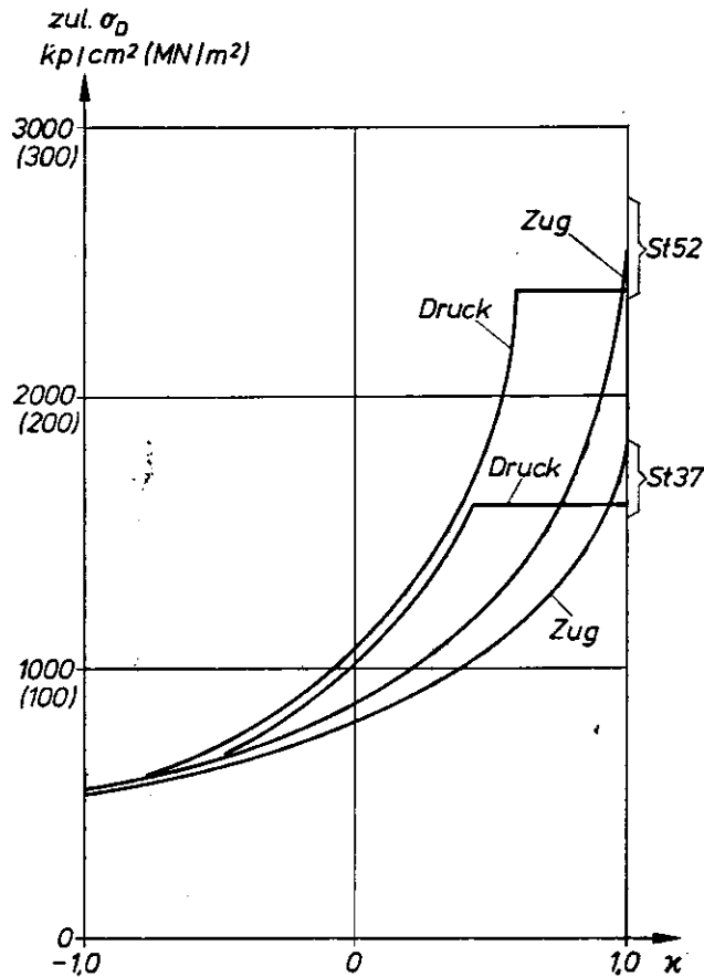
Bild 7. Zulässige Spannung für die Dauerfestigkeit; Kerbfall 3
