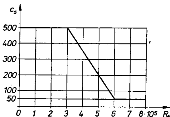
Bild 3. Beiwert c_s in Abhängigkeit von der Reynoldszahl
