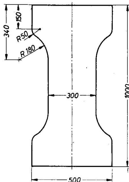
Bild 1. Probe für die Prüfung der Zugfestigkeit (zugleich Schablone zum Zuschneiden)
