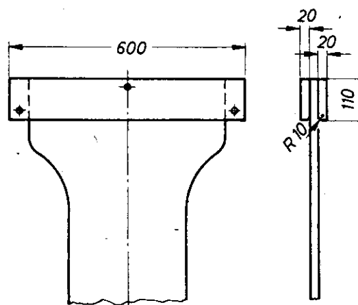
Bild 2. Einspannung der Probe nach Bild 1
