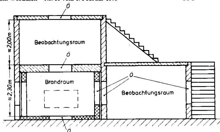
Bild 1. Längsschnitt Prüfstand
