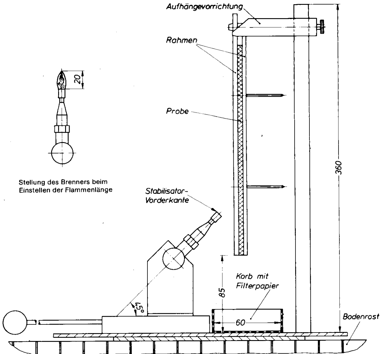
Bild 7. Anordnung (Prinzipdarstellung) zur Prüfung von Baustoffen der Klasse B 2
