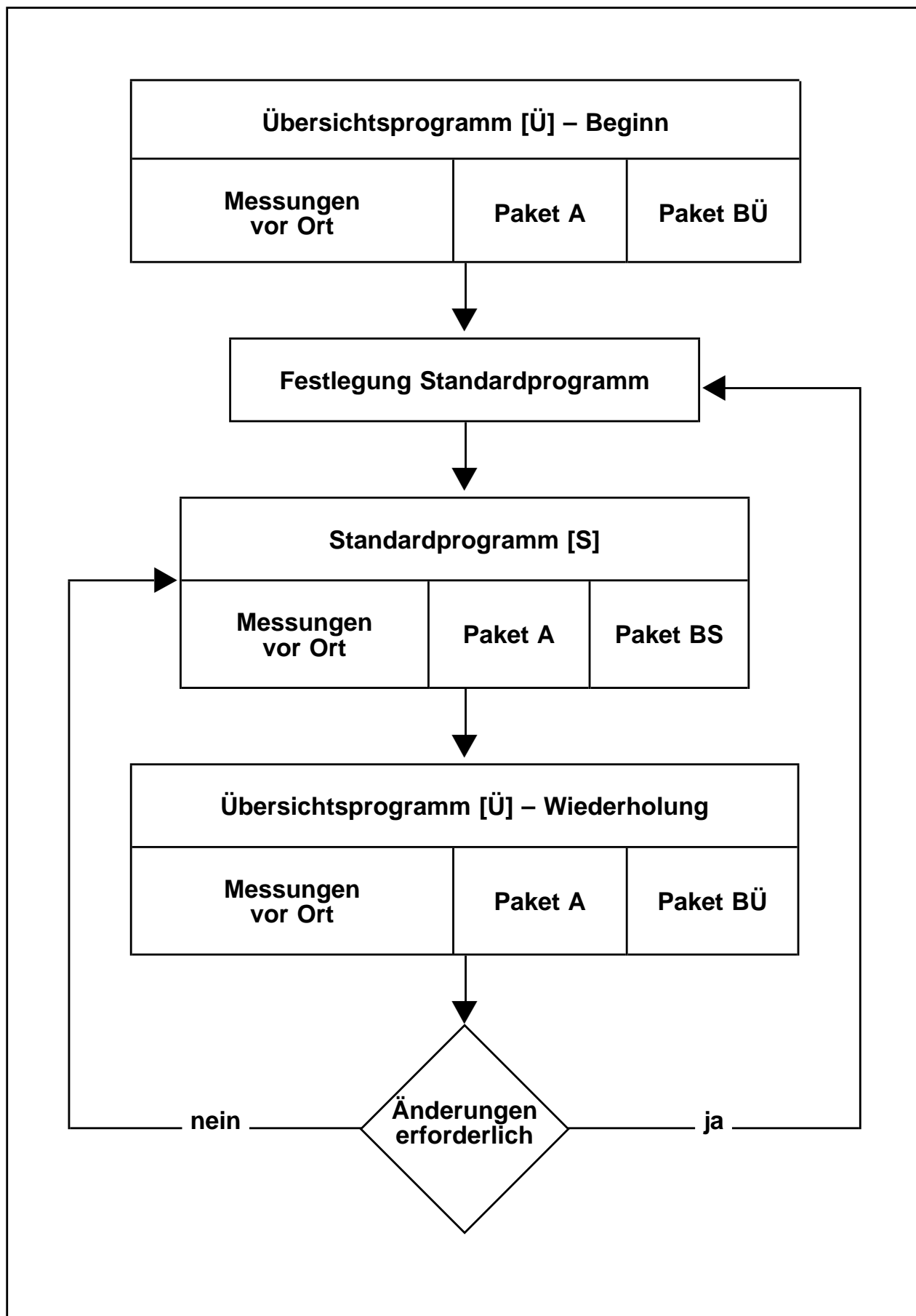
Abb. 1: Schematischer Ablauf der Sickerwasser- und Grundwasserüberwachung bei Deponien
